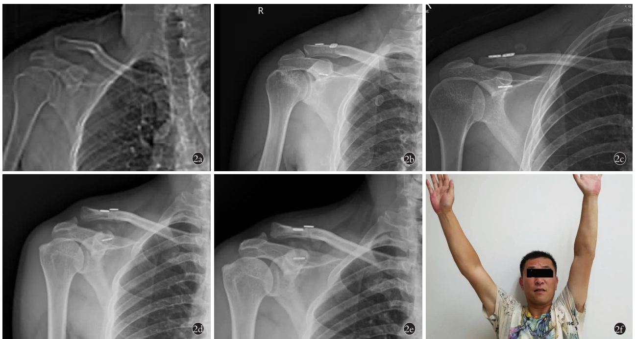
图 2 患者,男,50 岁,右侧肩锁关节脱位 Rockwood III 型 2a. 术前 X 线片示 Rockwood III 型损伤 2b. 术后 1 周 X 线片示锁骨远端低于肩峰,复位过度 2c. 术后 2 个月 X 线片显示肩锁关节复位有丢失 2d. 术后 5 个月 X 线片锁骨骨溶解并复位丢失 2e. 术后 8 个月 X 线片锁骨骨溶解并复位丢失 2f. 术后 12 个月右肩关节 Karlsson 功能评价为良
